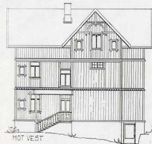
EKSISTERENDE FASADE
