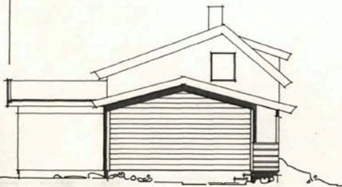
FASADE SØR
