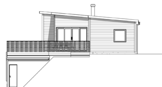
Fasade mot sør 1 : 100
