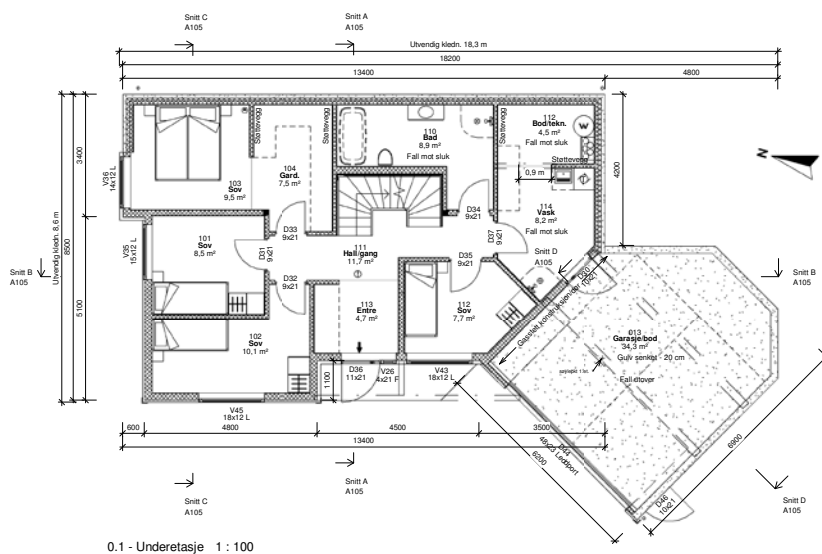
0.1 - Underetasje 1 : 100
