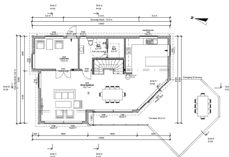
1.0 - 1. etasje 1 : 100
