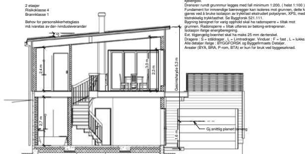
Snitt A 1 : 100
