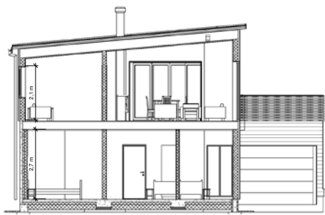
Snitt C 1 : 100
