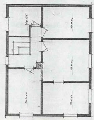
2. ETAGE
