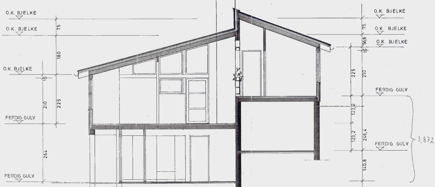
SNITT A-A
