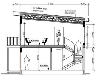
Snitt A-A
