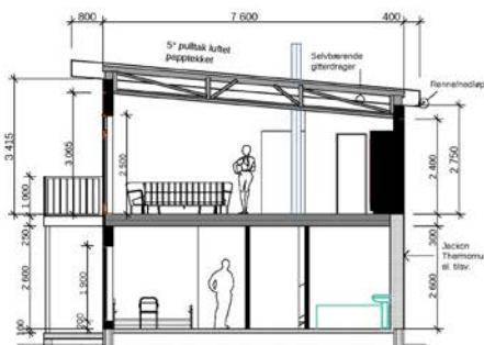
Snitt B-B
