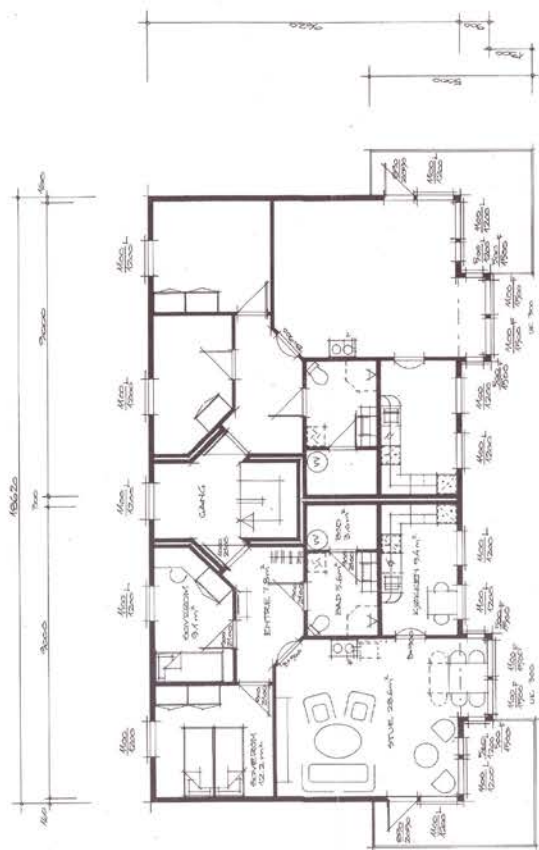
2. ETAGE
