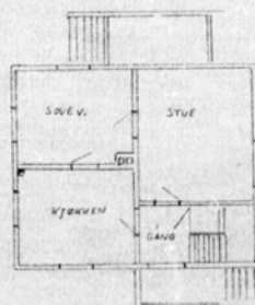
1. ETG. PLAN.
