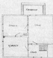
2. ETG. PLAN.
