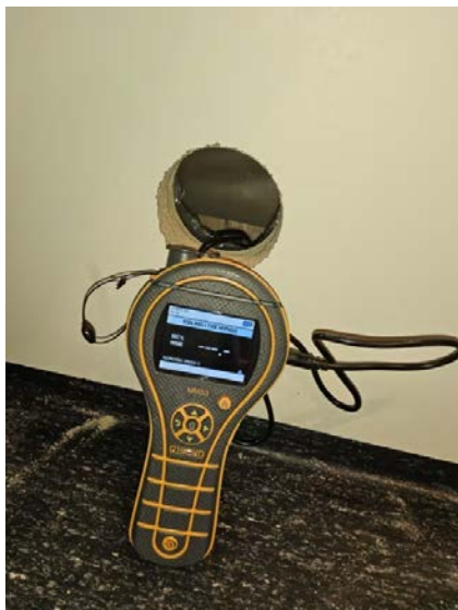
Bilde viser fuktmåling på vaskerom. Bilde viser plast i konstruksjonen.
