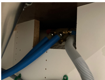
Plastrør inn mot bereder.
