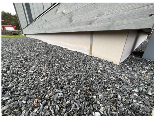
Utsnitt ringmurselementer.
