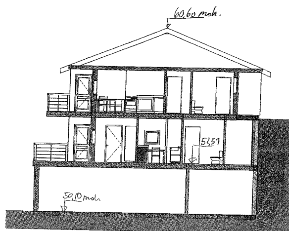
Snitt S-1
