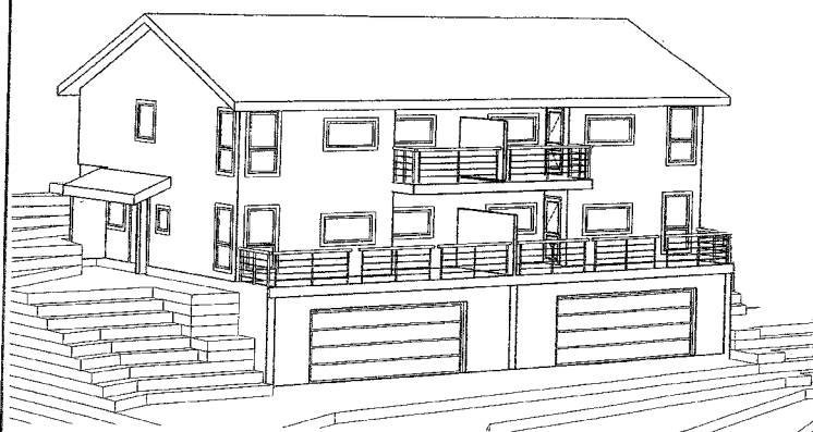
FRA SØR
