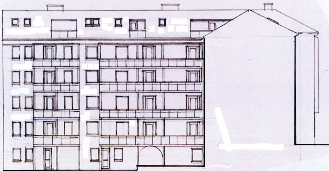
FASADE SØR mål. 1:200
