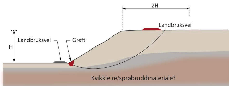
Figur 10 Graving og fylling i forbindelse med veibygging hvor det MÅ gjennomføres geotekniske vurderinger for vurdering av tilstrekkelig sikkerhet og gjennomførbarhet
