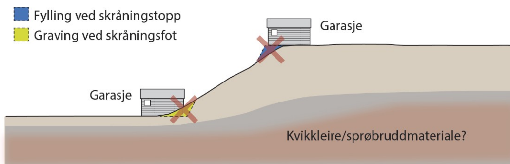
Figur 1 Graving og fylling hvor det MA gjennomføres geotekniske vurderinger for vurdering av tilstrekkelig sikkerhet og gjennomførbarhet
