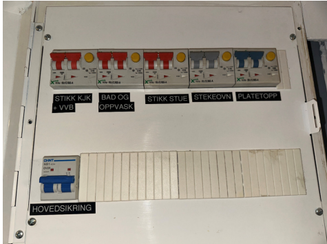
Sikringsskap med automatsikringer.
