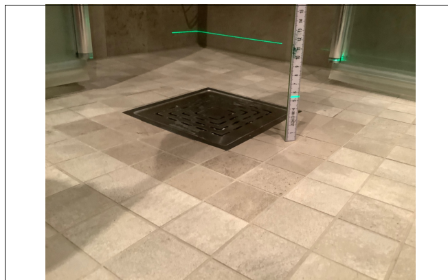
Kontroll av fall på gulv på våtrom.
