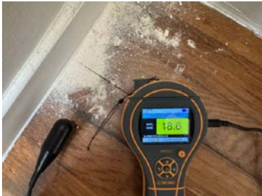
Fuktindikasjon på soverom i hybel del
