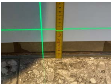
Fallforhold ca. 96 mm overkant gulv ved terskel
