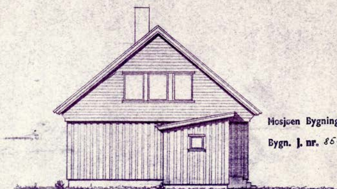
NORDØSTFASADE
