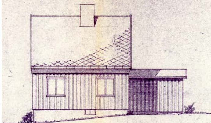
SYDØSTFASADE
