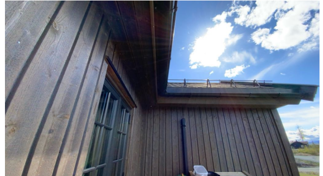
Synlige luftespalter i gesimskasse.
