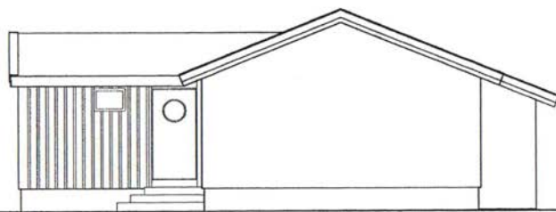
FASADE MOT SØR
