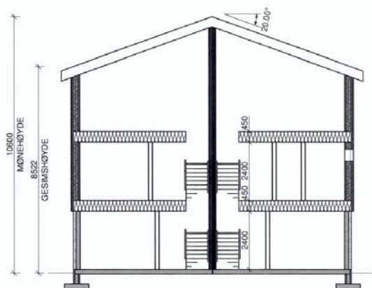
Snitt 1-1 1 : 100
