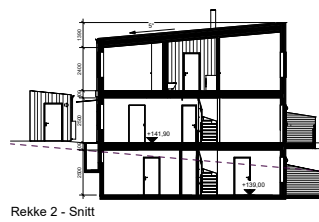
Rekke 2 - Snitt
