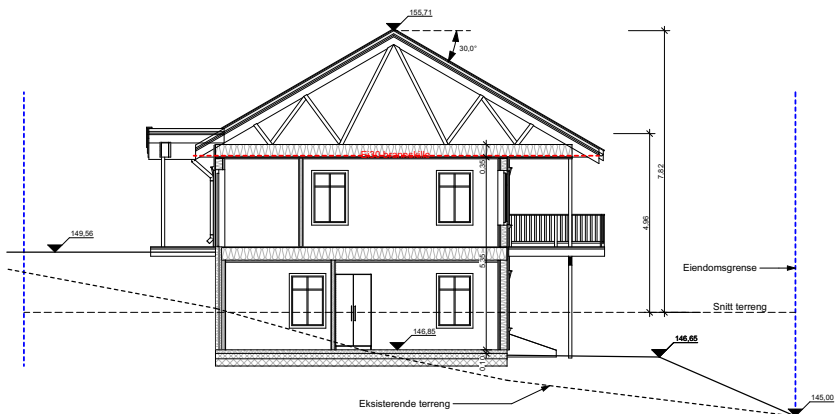
Snitt C
