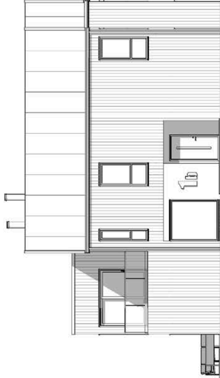
FASADE Ø
