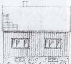
FASADE MOT SØRØST med Biermandsens vgl.
