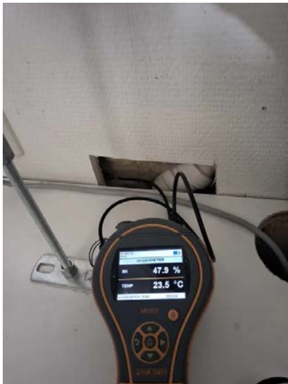
Bilde fra fuktmåling i veggkonstruksjon tilstøtende våtrom.
