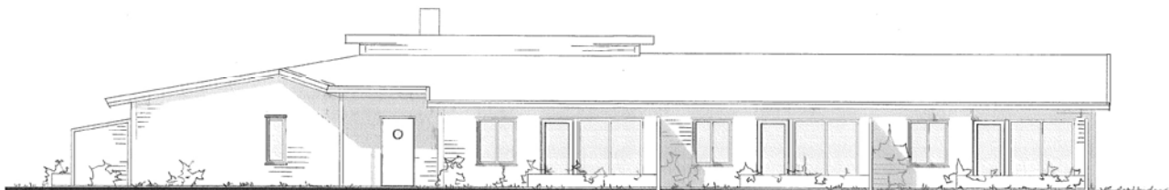
FASADE MOT SØR
