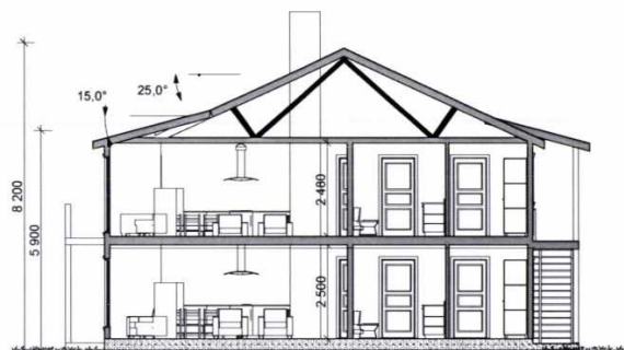
Snitt A-A
