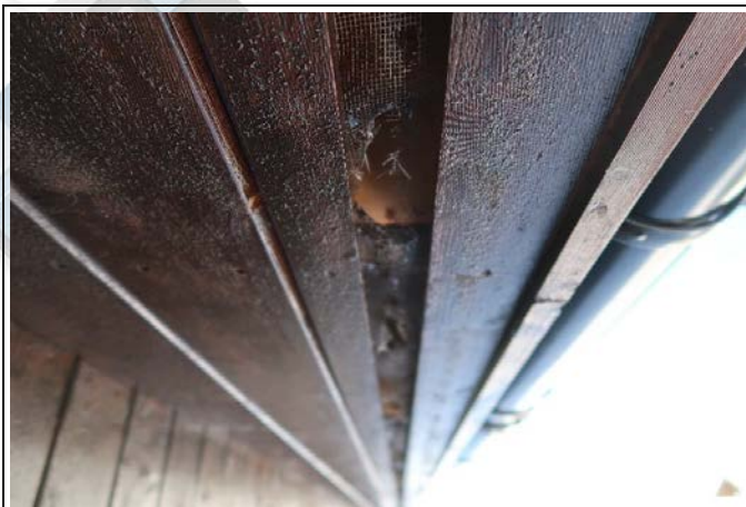
Eksempel på skadet fluenetting i luftespalte ved raft.
