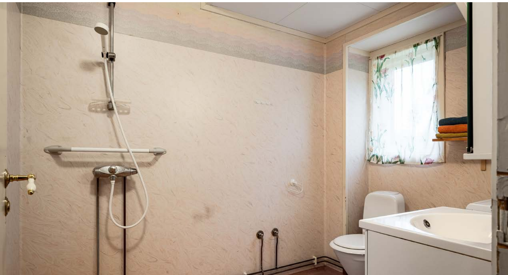
Eldre baderom fra ca. 1990 i 1. etasje. Badetrommet har belegg på gulv, elektrisk gulvvarme, våtromsbelegg på veggene og mekanisk ventilasjon med ventil på yttervegg.
