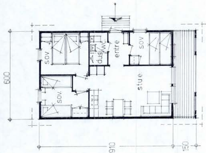
PLANLØSNING
