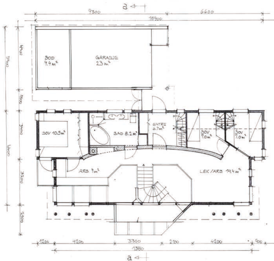
Plan 1.etasje Bruksareal: 91,56 m 2 Bebygd areal inkl. garasje: 148,59 m 2
