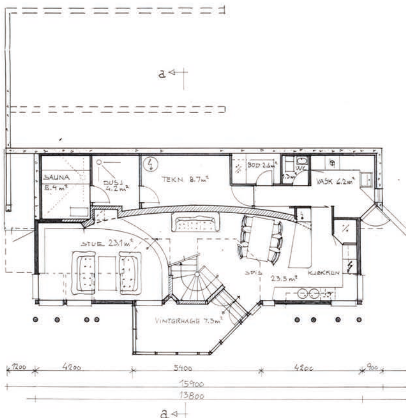
Plan under-etasje Bruksareal: 93,18 m 2 Bebygd areal, bolig: 109,20 m 2
