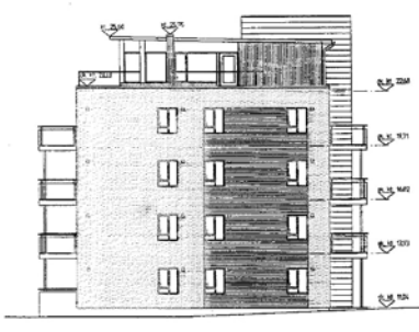
FASADE MOT SØR
