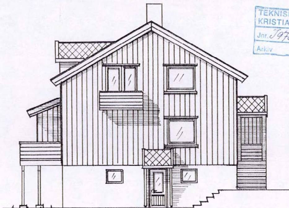
FASADE ØST.
