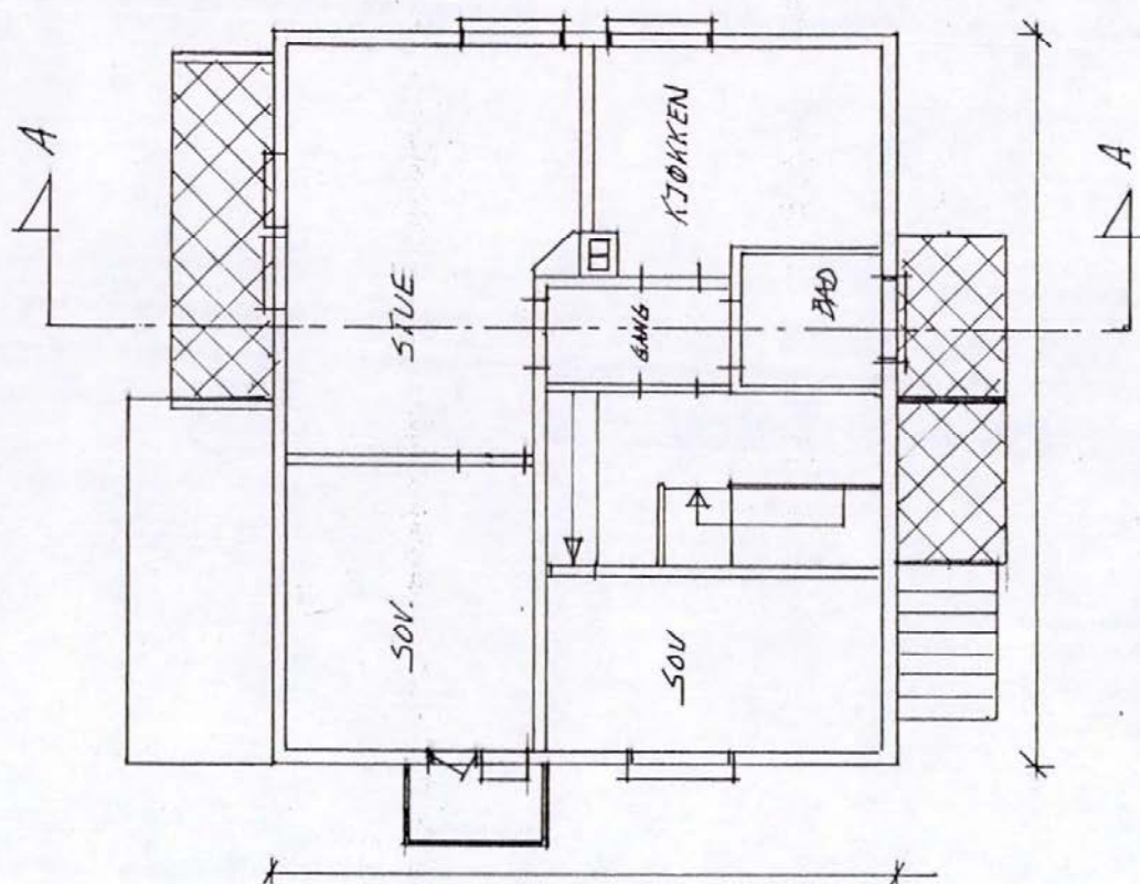
PLAN 2. ETG.
