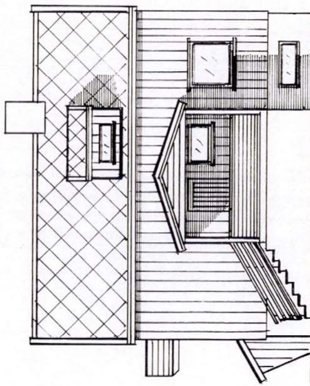
FASADE NORD.
