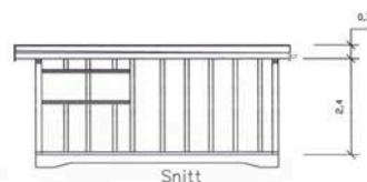
Snitt
