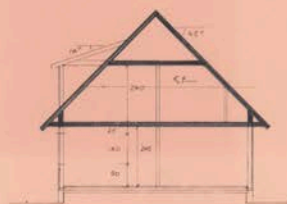
SNITT
