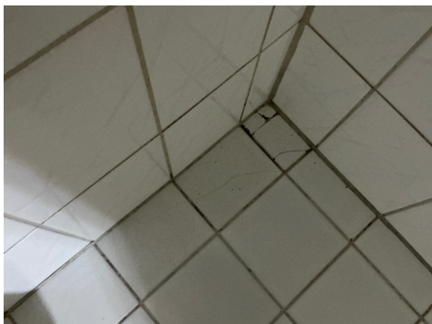
Riss i fliser i våtsonen
