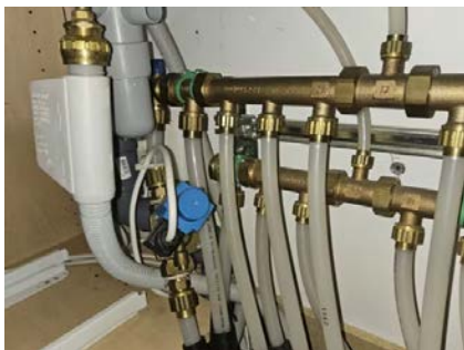
Åpen rørfordeling med automatisk vannstoppeventil under kjøkkenvask.
