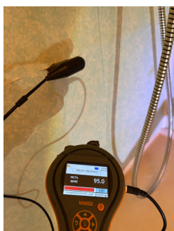
Skade på våtromsplate i dusjsonen.
