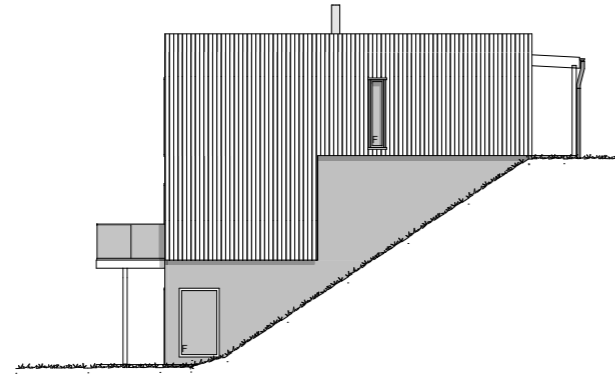
Fasade Nord-Øst FG=186.3 MOH
