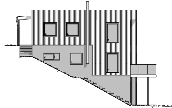
Fasade Sør-Vest FG=186.3 MOH
