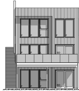
Fasade Sør-Øst FG=186.3 MOH
