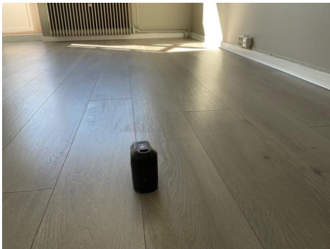
Nivellering stue/kjøkken, avvik ca. 10-20 mm
