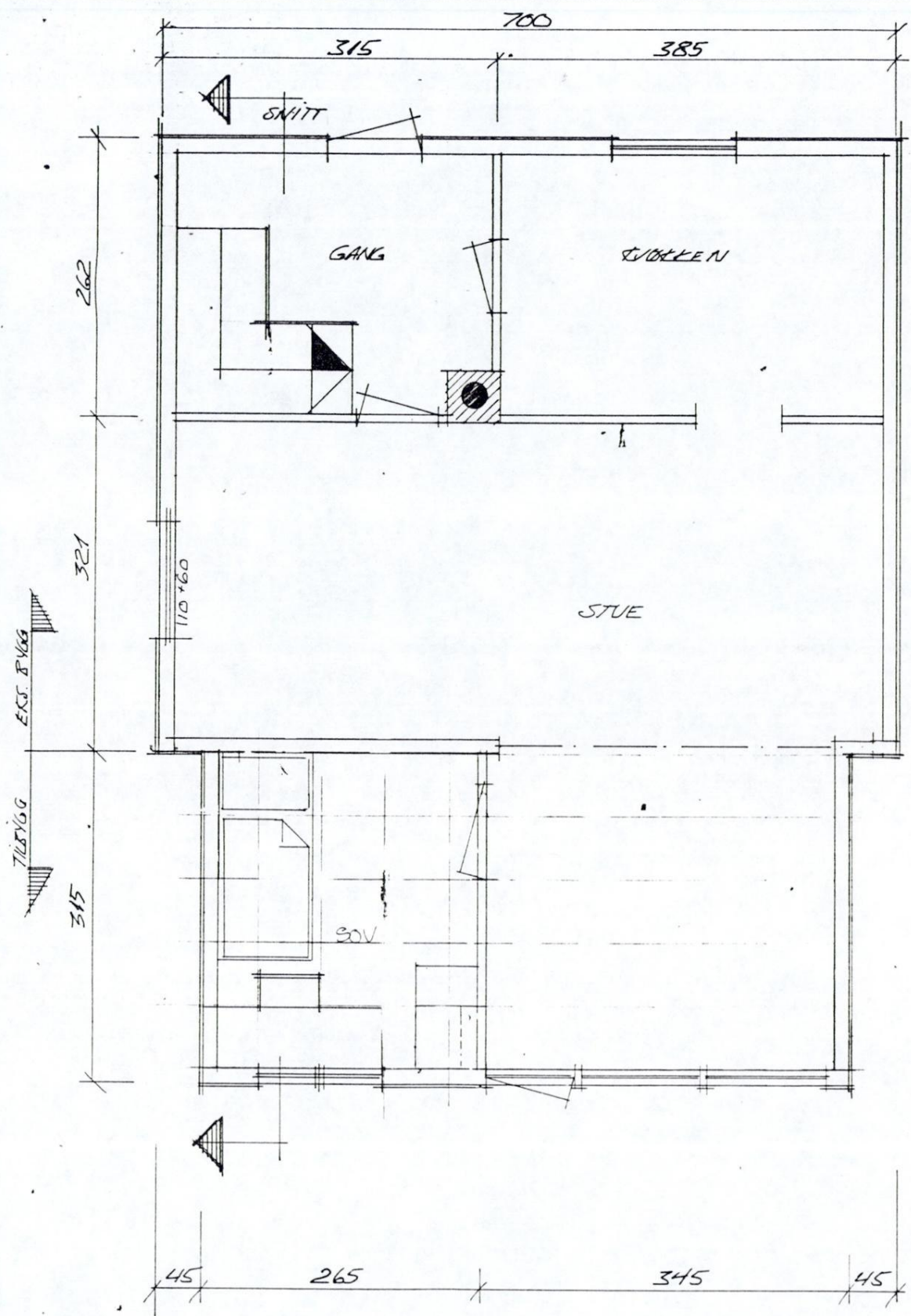
PLAN 1:50
