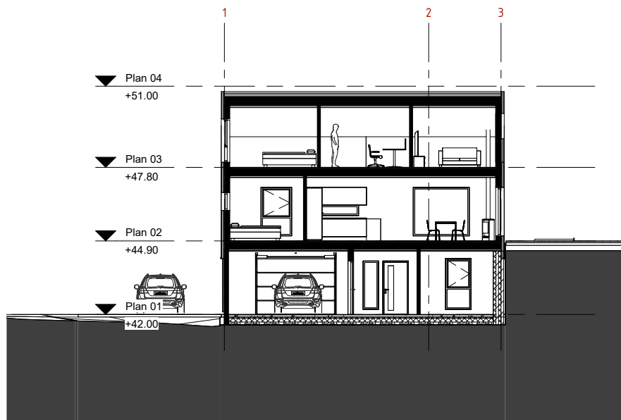
SNITT B-B 1 : 100
