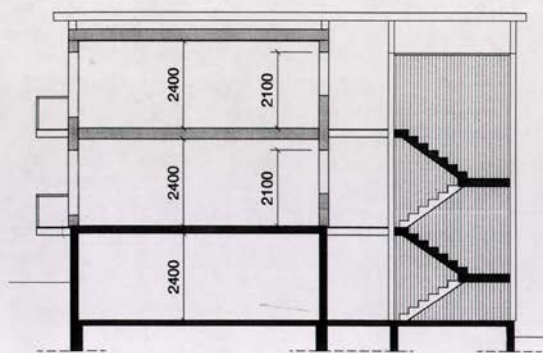
SNITT C - C
