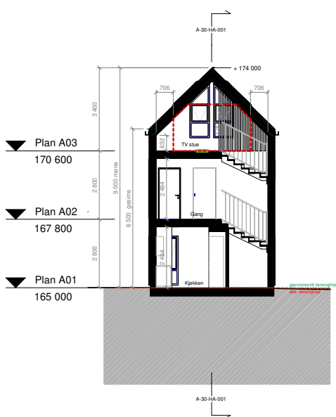
Snitt A1 1 : 100
