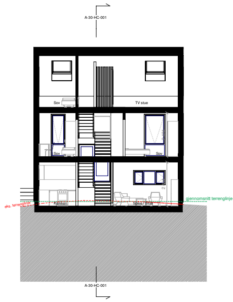
Snitt C2 1 : 100
