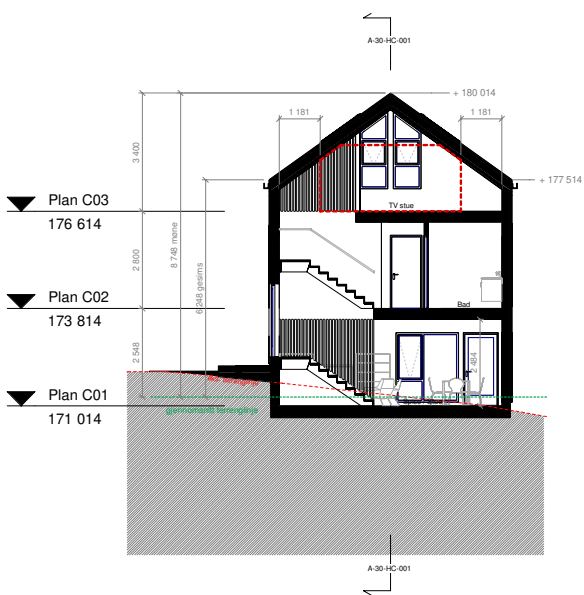
Snitt C1 1 : 100
