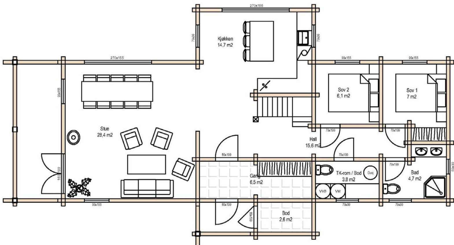
Planskisse 1. etasje
