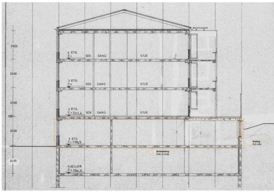
Ole Reistads vei 1 B / Snitt 01
