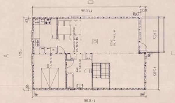
PLAN 1. ETG.
