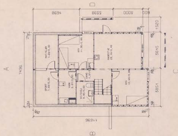
PLAN SOKKEL
