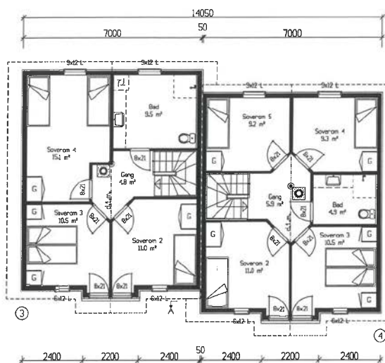
PLAN 2. ETASJE Garderobeskapene må plassbygges
