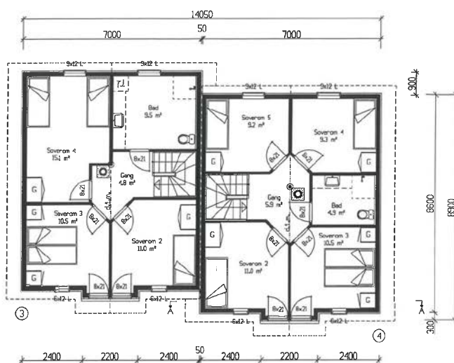
PLAN 2. ETASJE Garderobeskapene må plassbygges
